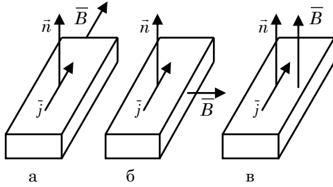
Рис. 1 – Взаємна орієнтація векторів \vec{B} , \vec{j} та \vec{n} при геометріях вимірювання: повздовжній МО (а), поперечний (б) та перпендикулярній (в)
