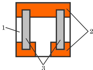
Рис. 4 – Схематичне зображення ПО для демонстрації і вивчення явища гігантського магнітоопору: 1 – скляна підкладка; 2 – контактні площадки; 3 – плівковий резистор
