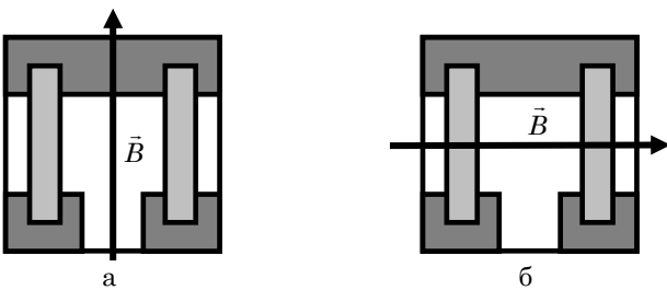
Рис. 7 – Розташування плівкового об’єкта в області магнітного поля: а – вимірювання повздовжнього магнітоопору ( R_{||} ); б – вимірювання поперечного магнітоопору ( R_{\perp} )
