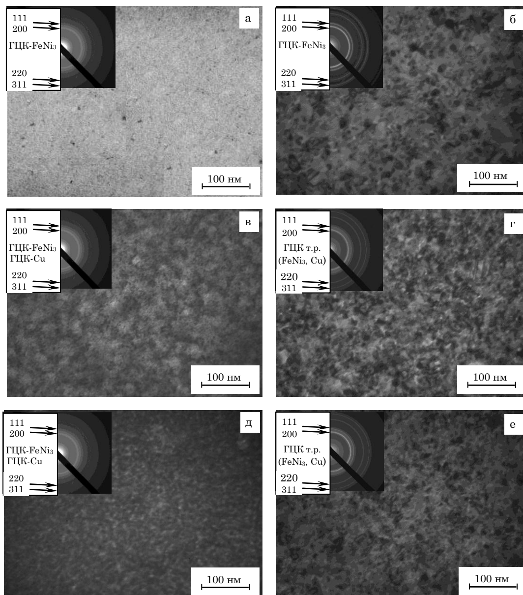
Рис. 1 – Мікроструктура одношарових плівок пермалою (а, б) та тришарових плівкових структур Py/Cu/Py (в-е) у свіжосконденсованому (а, в, д) та відпаленому за температури 700 К (б, г, е) стані (а, б – d_{Py} = 40 нм; в, г – 2d_{Py} = 60 нм, d_{Cu} = 7 нм; д, е – 2d_{Py} = 80 нм, d_{Cu} = 5 нм). На вставках наведені відповідні електронограми
