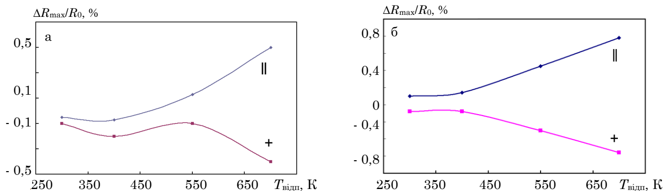
Рис. 4 – Залежність \Delta R_{\max}/R_0 від температури відпалювання для тришарових плівок \text{Pu}/\text{Cu}/\text{Pu} з товщинами шарів а – d_{\text{Pu}} = 30 нм, d_{\text{Cu}} = 7 нм; б – d_{\text{Pu}} = 50 нм, d_{\text{Cu}} = 5 нм
