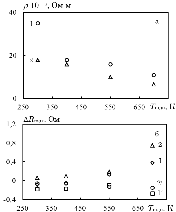
Рис. 3 – Залежність питомого опору \rho (а) та величини \Delta R_{\text{max}} (б) від температури відпалювання для тришарових плівок \text{Ru}/\text{Cu}/\text{Ru} з товщинами шарів 1 - d_{\text{Ru}} = 30 нм, d_{\text{Cu}} = 7 нм; 2 - d_{\text{Ru}} = 50 нм, d_{\text{Cu}} = 5 нм
