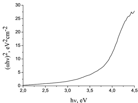
Рис. 4 – Залежність (\alpha \cdot hv)^2 від енергії фотона h\nu
