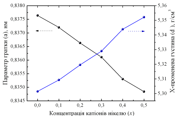
Рис. 4 – Залежність параметра ґратки і густини d_x кілець від Ni^{2+}
