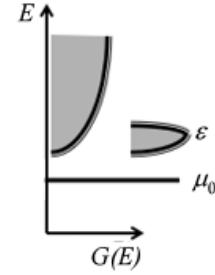
Рис. 11 – К проектированию наилучших термоэлектриков
