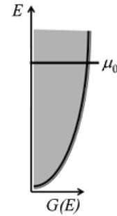
Рис. 12 – К увеличению проводимости термоэлектрика
