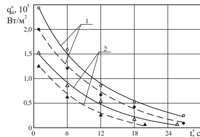
Рис. 6 – Залежності q_n^*(t^*) для елементів з оптичного скла ТФ110 (1) та БК10 (2) (товщина елемента H = 4 \cdot 10^{-3} м: ——— P = 10^5 Па; - - - - - P = 10^7 Па; ●, ○, ▲ – експериментальні дані
