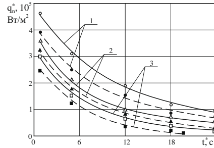
Рис. 5 – Залежності q_n^*(t^*) для елементів з оптичного скла К8 (1), К208 (2) та К108 (3) (товщина елемента H = 4 \cdot 10^{-3} м): ——— P = 10^5 Па; - - - - - P = 10^7 Па; ●, ○, ▲, □, ■ – експериментальні дані
